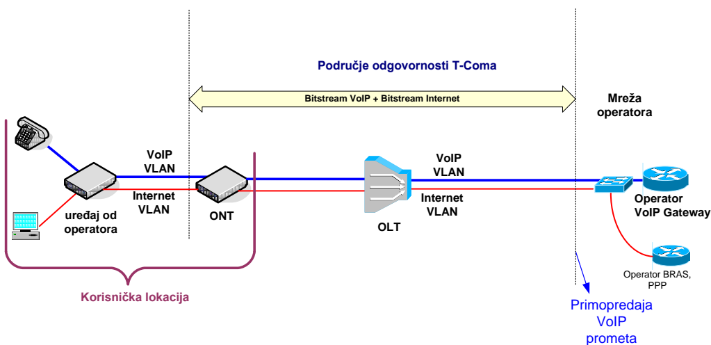
Slika 18. Veleprodajni širokopojasni pristup za pružanje VoIP usluge preko FTTH pristupa (GPON) na OLT razini
