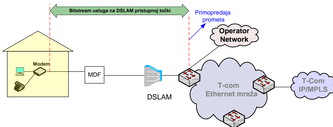
Slika 7. Veleprodajni širokopoljasni pristup za pružanje Internet usluge na DSLAM razini u slučaju kada krajnji korisnik ostvaruje Osnovni pristup mreži putem usluge HT-a
